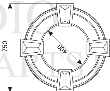
Dekor DA4 profil AS104 + zworniki AS128
