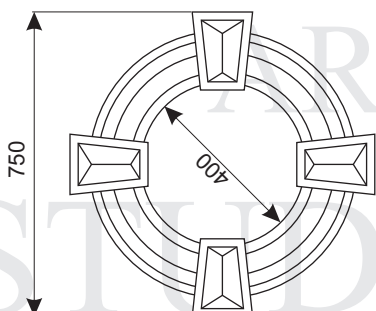
Dekor DA2 profil AS1 + zworniki AS128
