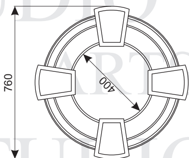
Dekor DA3 profil AS104 + zworniki AS93
